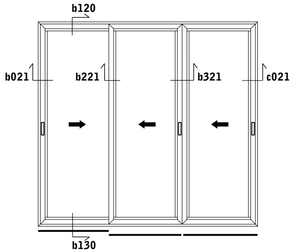
PERFIL DE CRUCE NT71-2160 (12132): H-73,2
