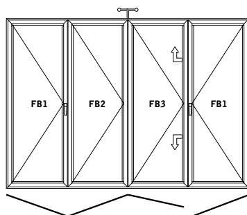
P500D1 (4+1)
