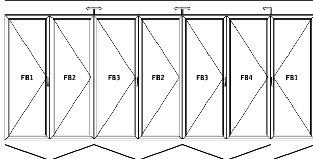
P700D3 (4+3)
