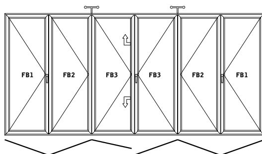
P700D1 (6+1)
