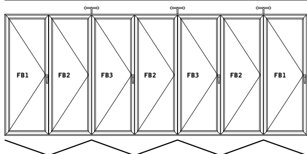
P700D2 (5+2)
