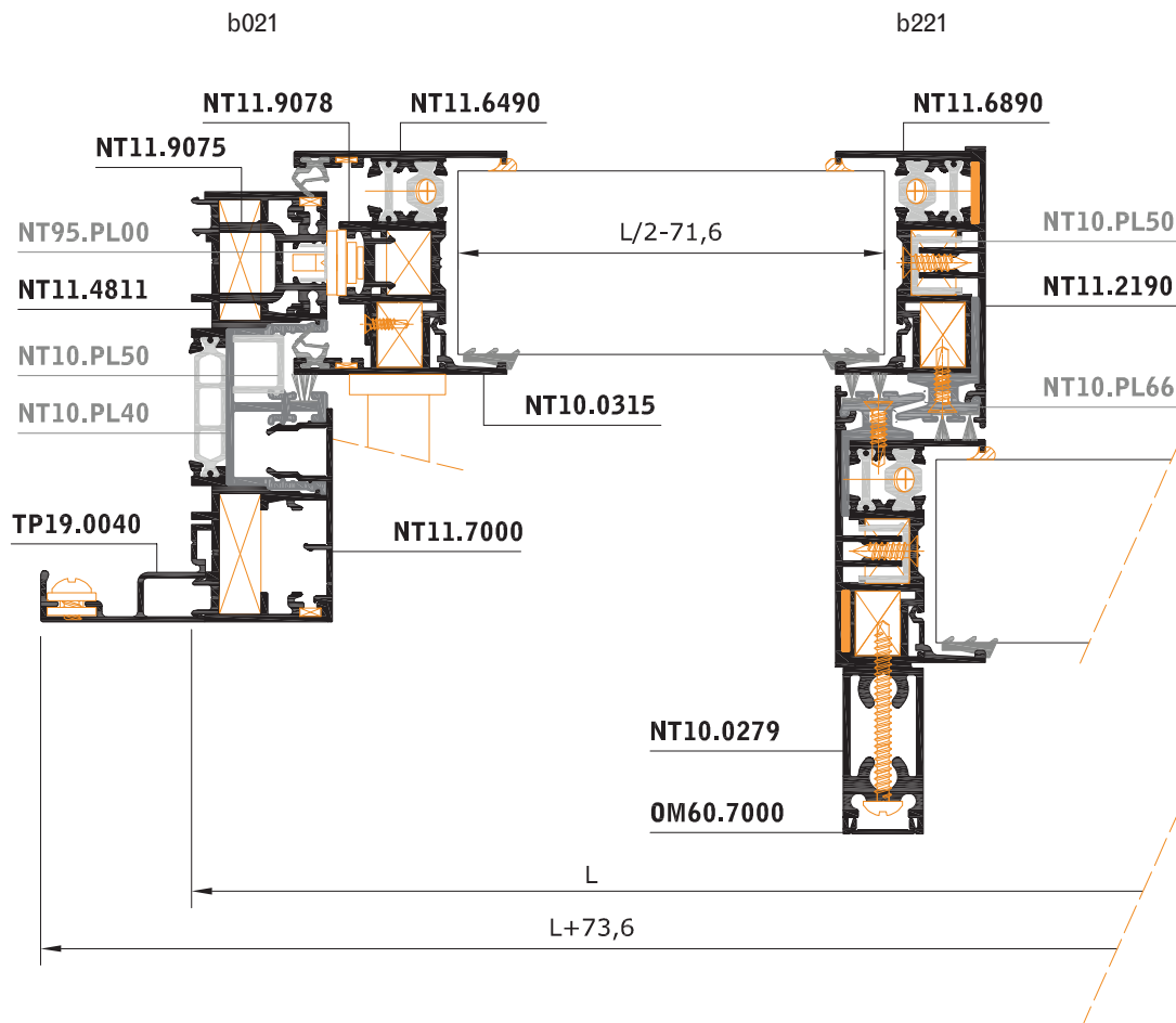
SECCIÓN HORIZONTAL b021-b221
