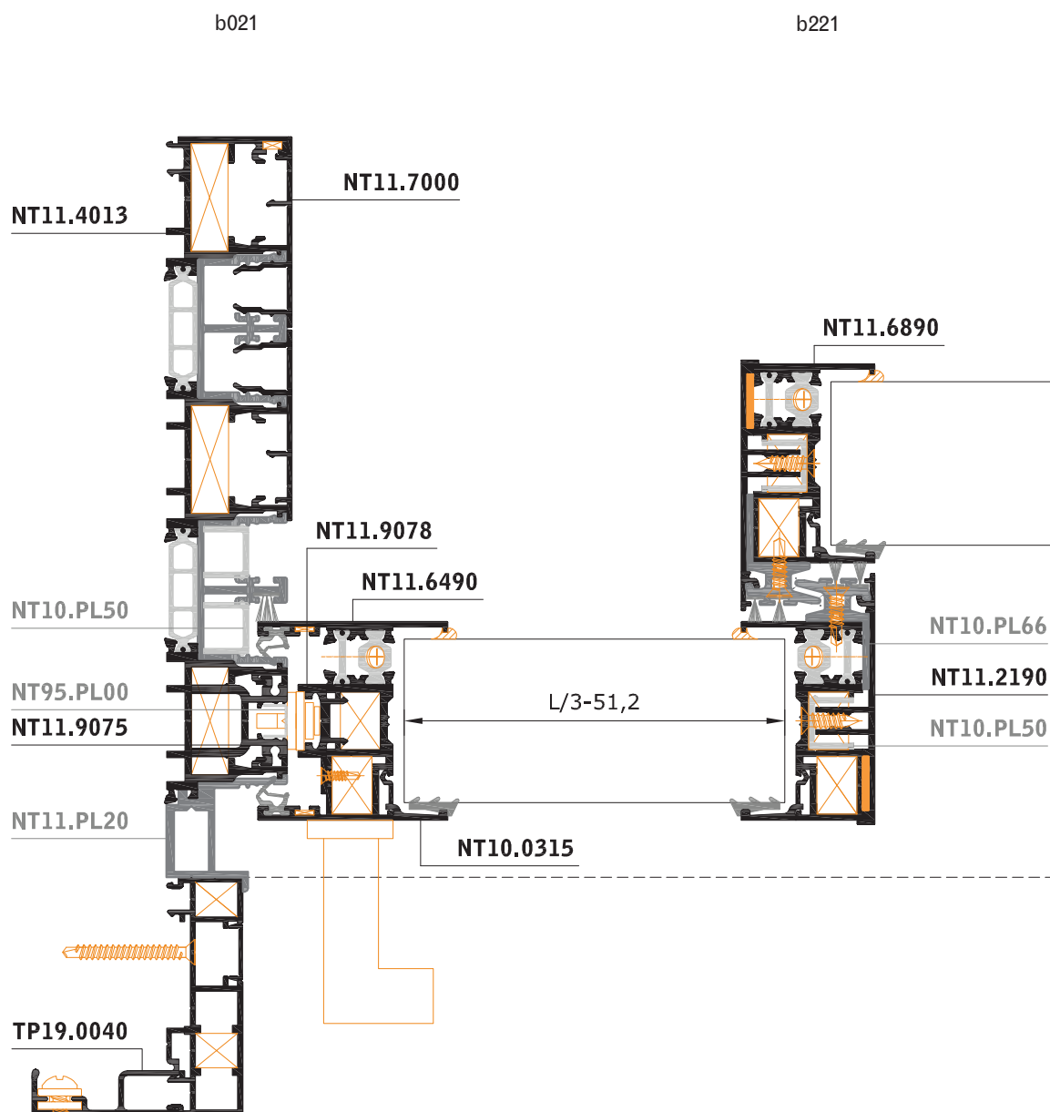
SECCIÓN HORIZONTAL b021-b221-b321-b421-c021
