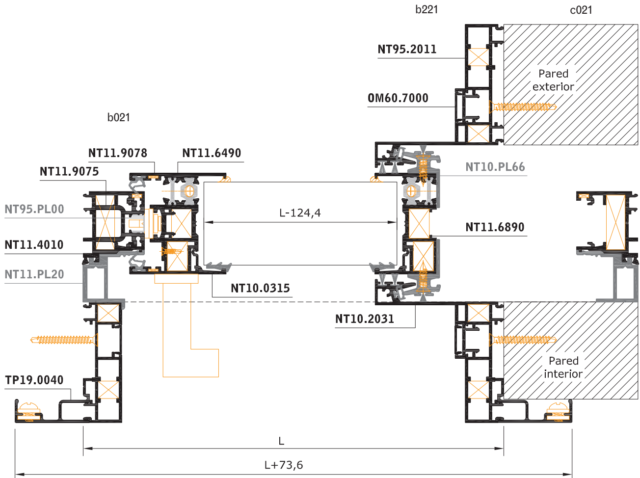
SECCIÓN HORIZONTAL b021-b221-c021
